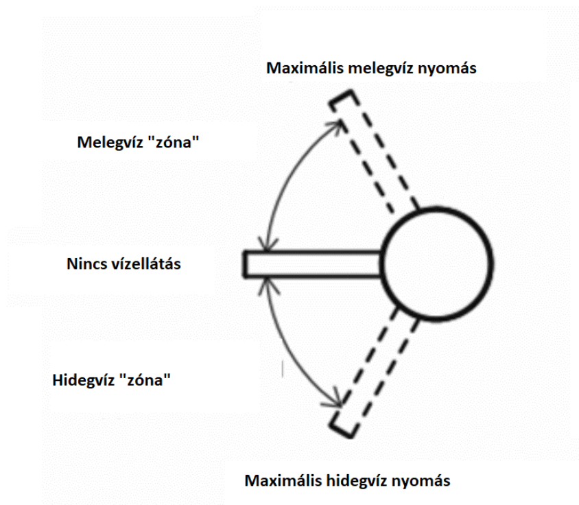
3. ábra A maximális vízhozam szabályozása.
