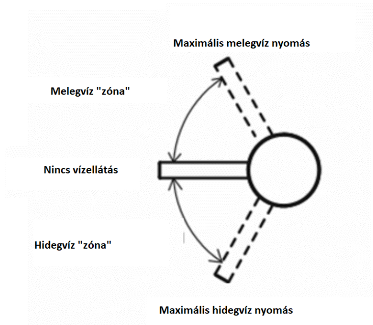
3. ábra A maximális vízhozam szabályozása.
