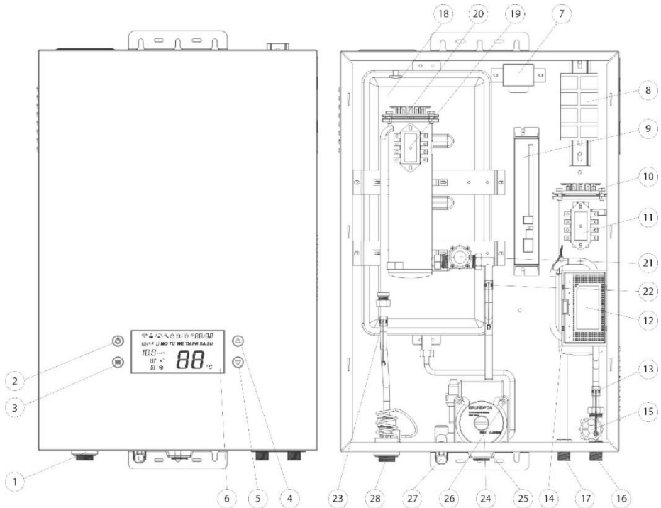
Ábra 1. kazán részegységek
