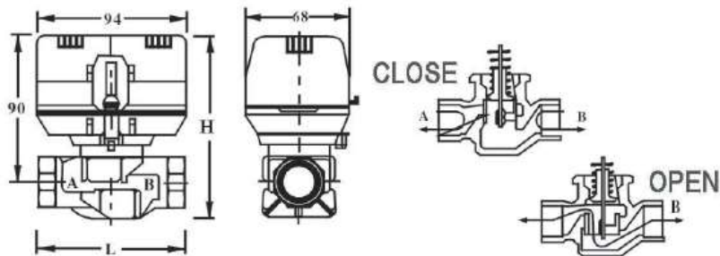
2. ábra: Két utas váltószelep műszaki rajza
