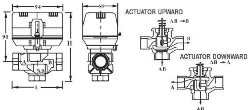
3. ábra: Három utas váltószelep műszaki rajza
