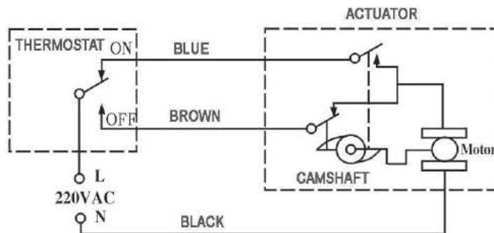
4. ábra: Kapcsolási rajz
