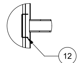
DETAIL AI SCALE 1 : 10
